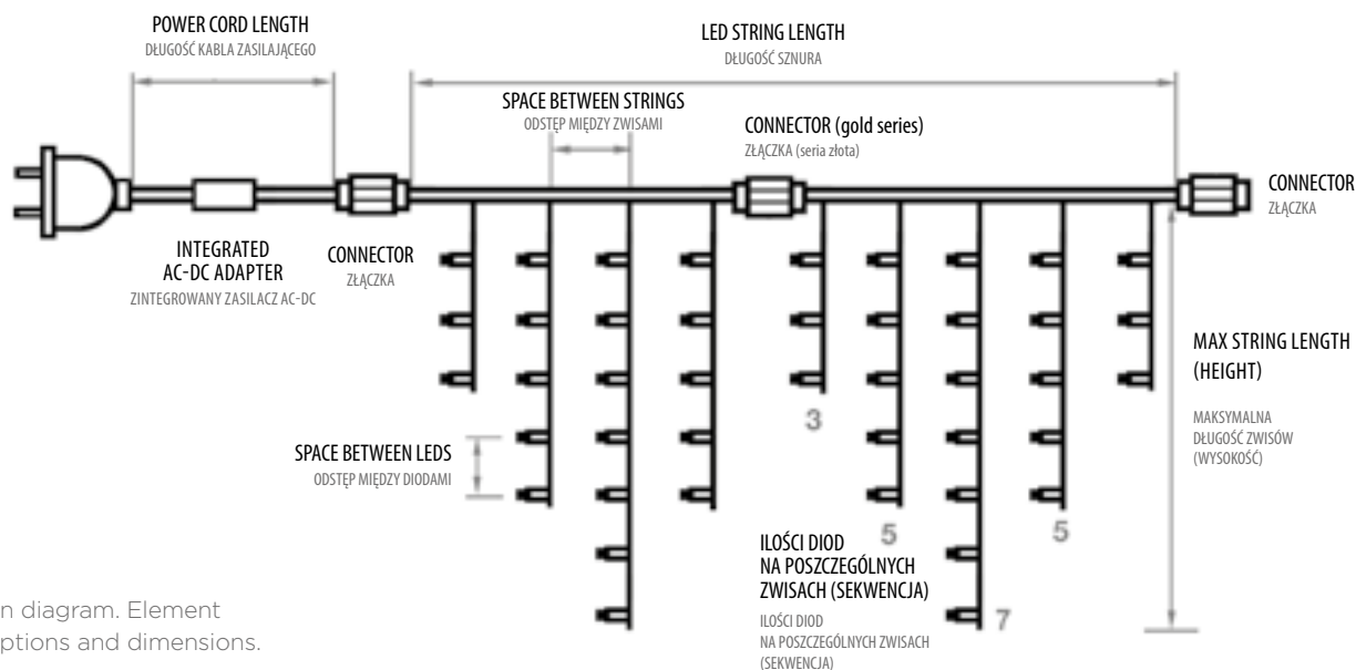
Schemat kurtyнки. Opisy elementów i wymiarowań.
